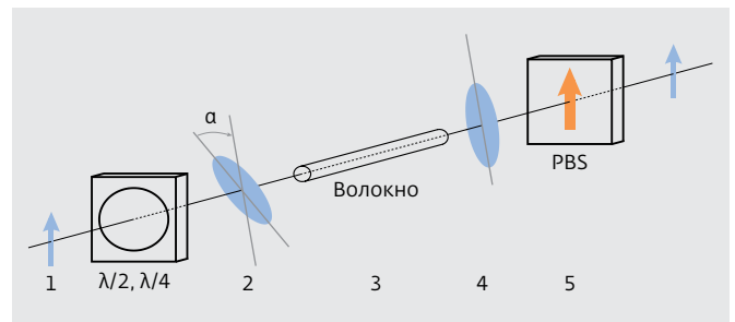
Рис.1. Схема насыщающегося поглотителя на основе эффекта НЭП. 1, 5 – линейное состояние поляризации на входе и выходе из системы, \lambda/2 , \lambda/4 – двулучепреломляющие пластинки, 2, 4 – эллипсы поляризации на входе и выходе из волокна, \alpha – угол поворота эллипса поляризации в волокне, 3 – волокно, 5 – поляризационный делитель
